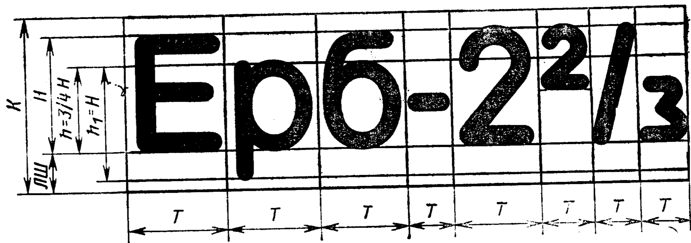
H — высота шрифта; K — высота площадки ( \frac{3}{2} H ), T — ширина площадки; ЛШ — расстояние от основания площадки до линии шрифта ( \frac{1}{2} H )
