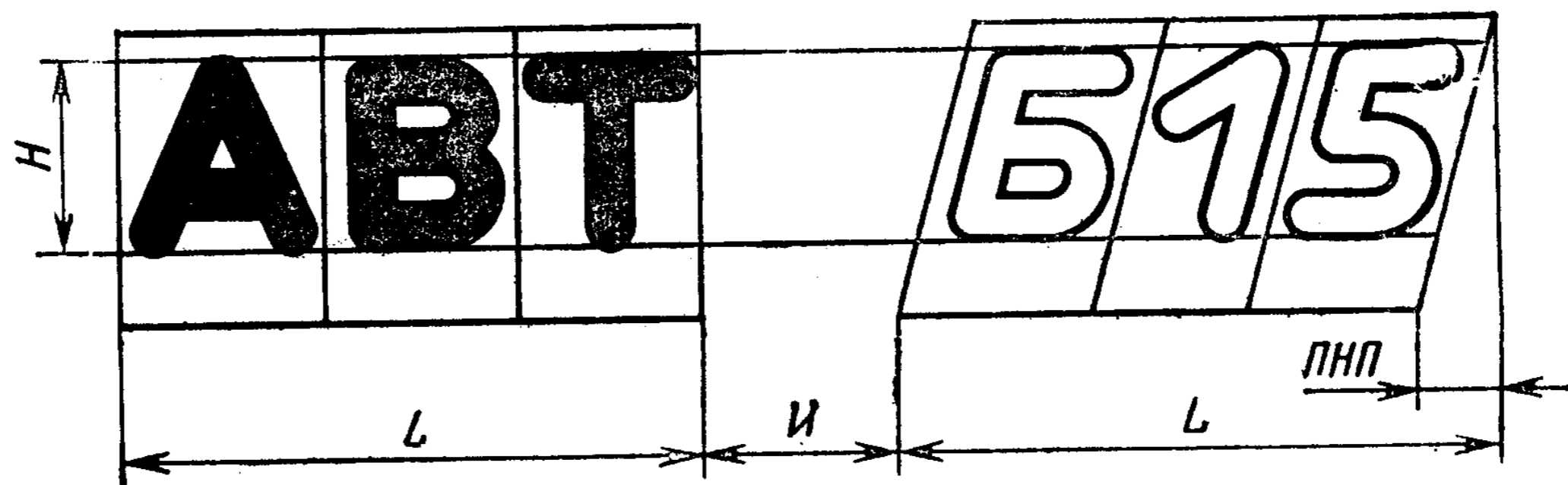
ПНП — проекция боковой стороны наклонной площадки; И — расстояние между надписями; L — длина надписи
